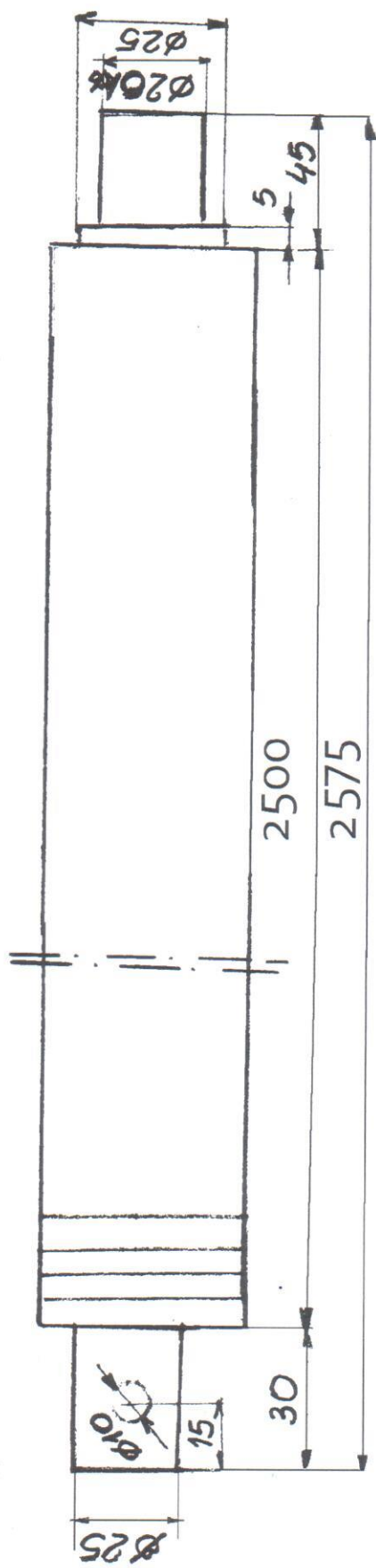
GWINT TRAPEZOWY 44 x 7 -prawy -lewy
